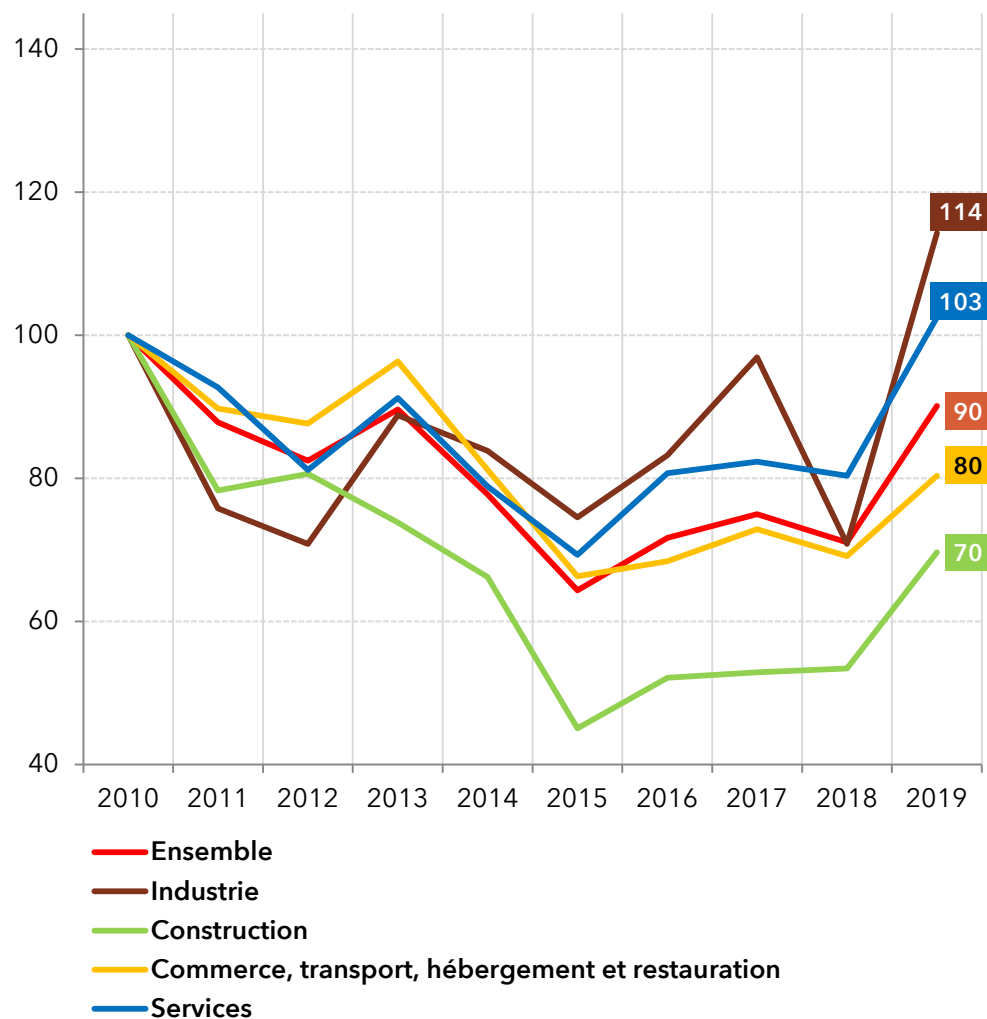
INDICE BASE 100 EN 2010 - ARDENNES
